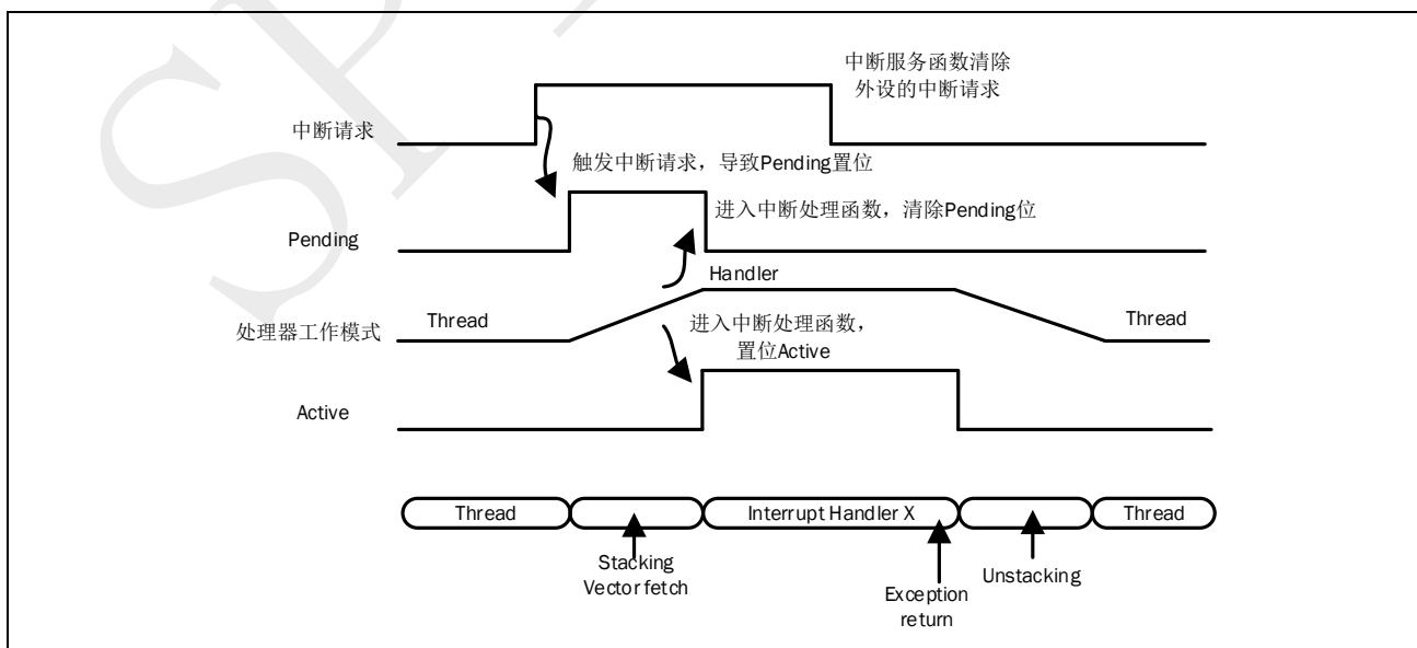
图 3-1: 中断状态的时序简图
