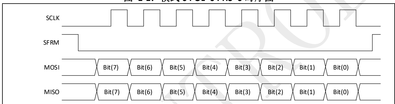
图 1-1: 模式 0 POL=0 PHS=0 时序图
