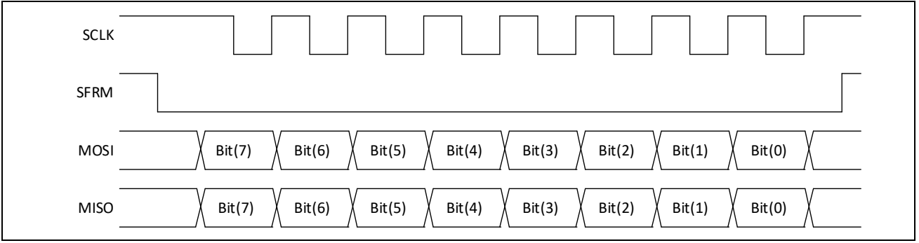
图 1-3: 模式 2 POL=1 PHS=0 时序图
