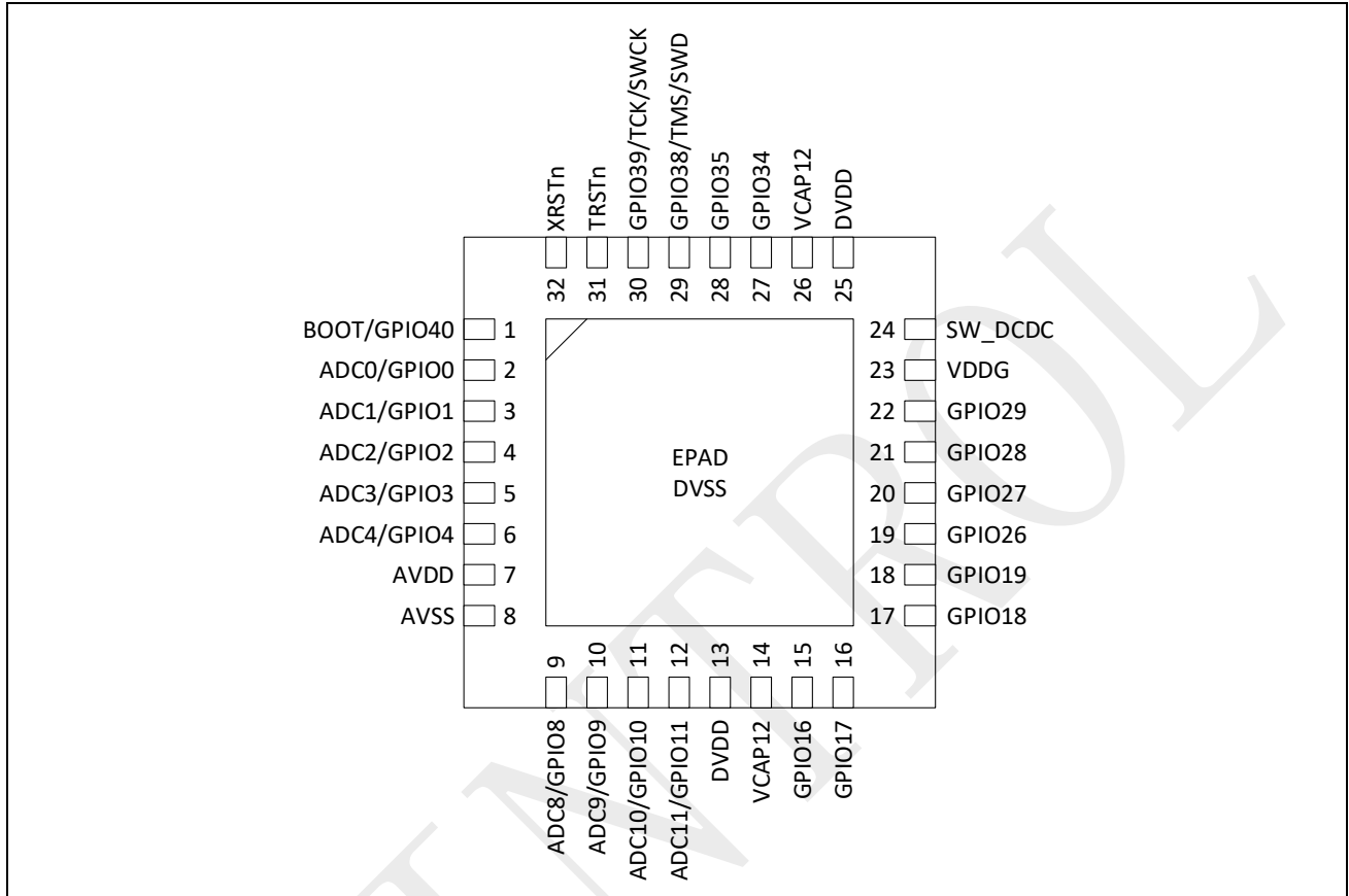
图 3-2: SPC1158 QFN32 引脚排列
