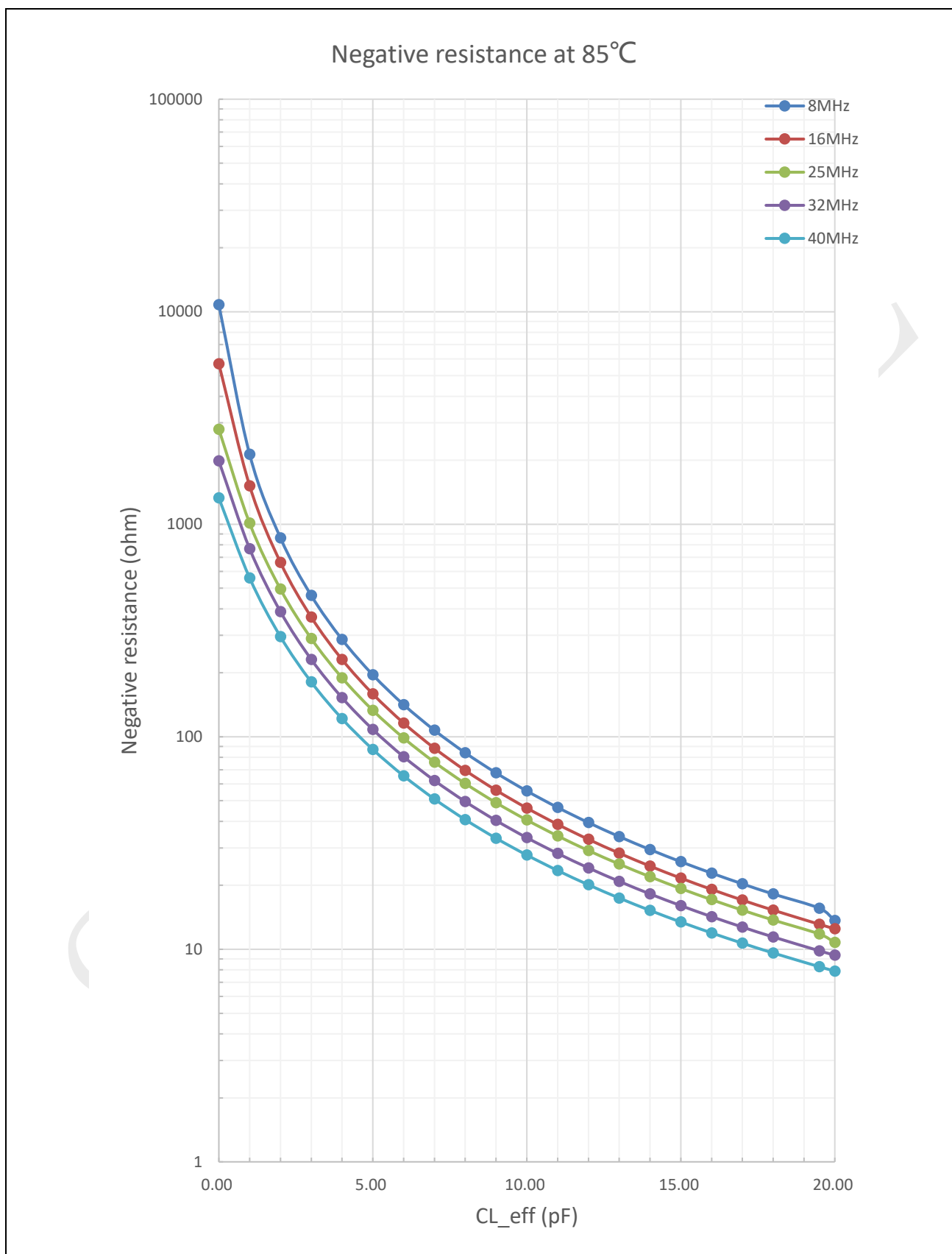
图 5-7: 内部晶振负阻值 (85°C)
