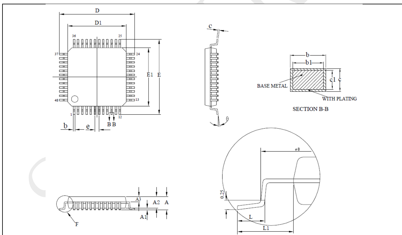
图 7-1: LQFP48 – 48 脚, 7 x 7 mm 薄型正方扁平封装图
