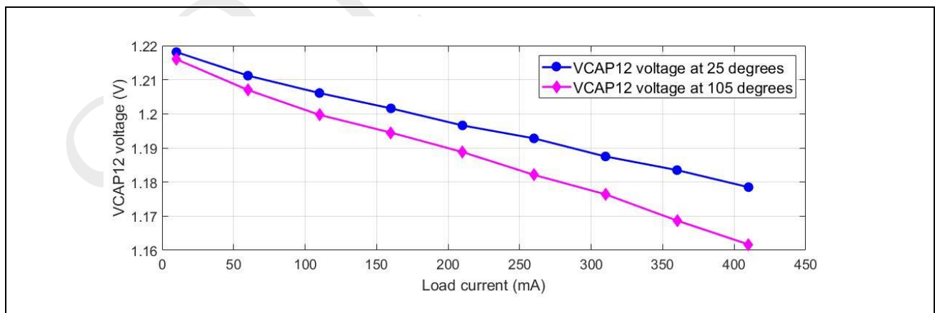
图 5-5: 内部 1.2V 稳压器负载调节率随温度变化情况
