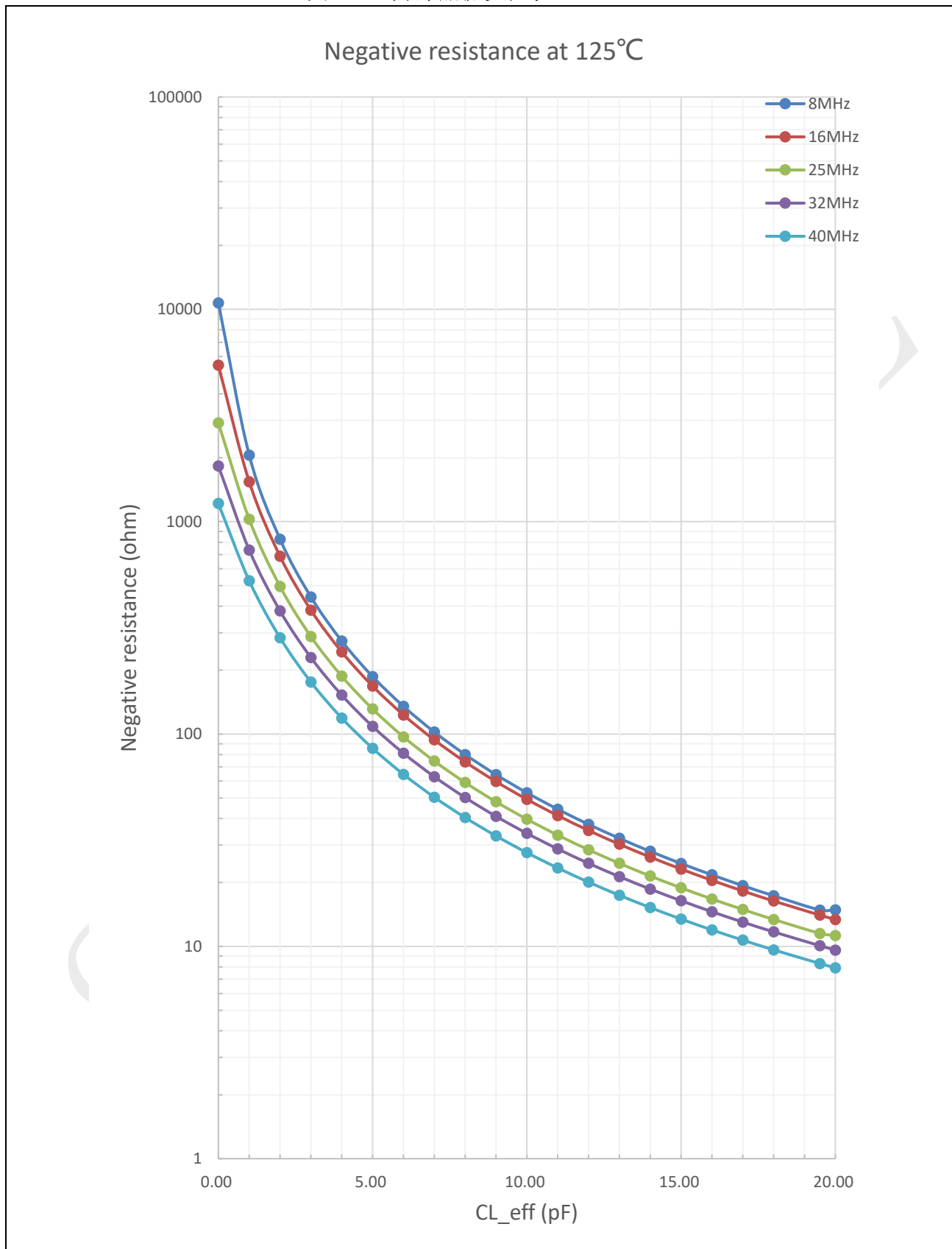
图 5-9: 内部晶振负阻值 (125°C)
