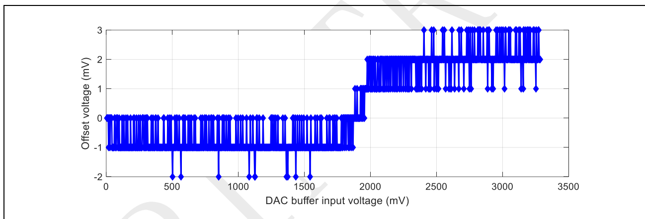
图 5-10: 数模转换器缓冲器偏移电压随输入电压变化关系
