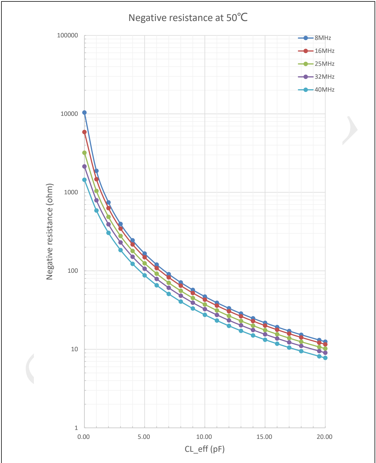
图 5-6: 内部晶振负阻值 (50°C)
