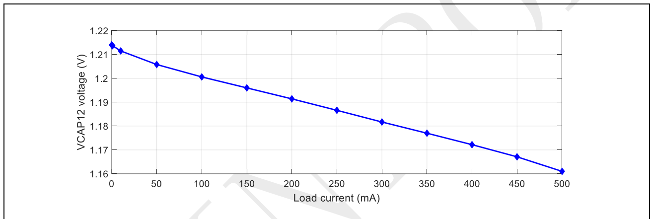
图 5-4: 内部 1.2V 稳压器负载调节率 ( T_A = 25^\circ\text{C} )
