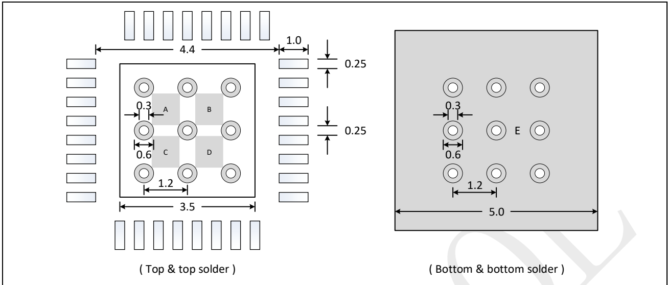
图 7-4: QFN32 – 32 脚, 5 x 5 mm 方形扁平无引脚封装推荐尺寸
