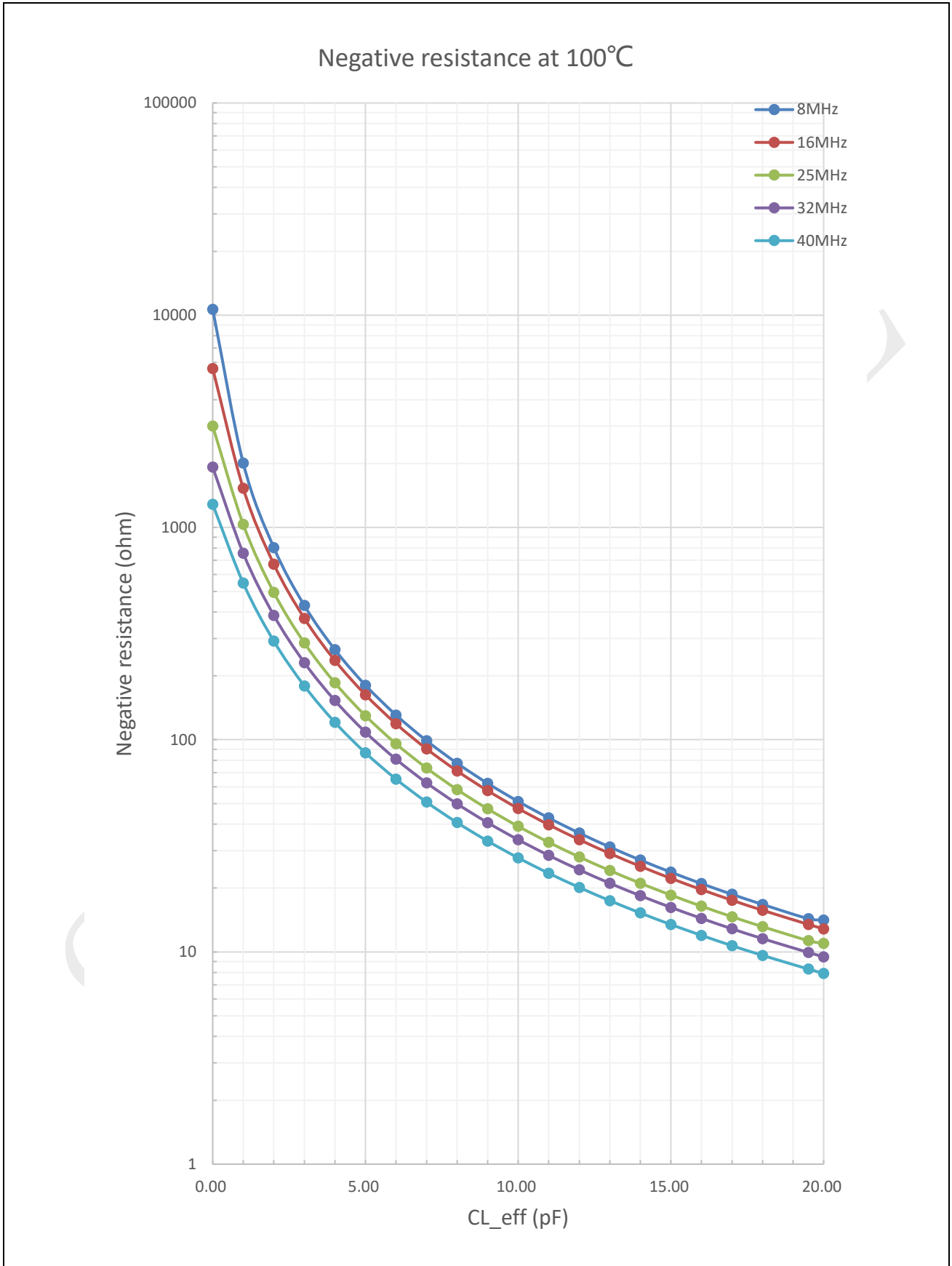
图 5-8: 内部晶振负阻值 (100°C)
