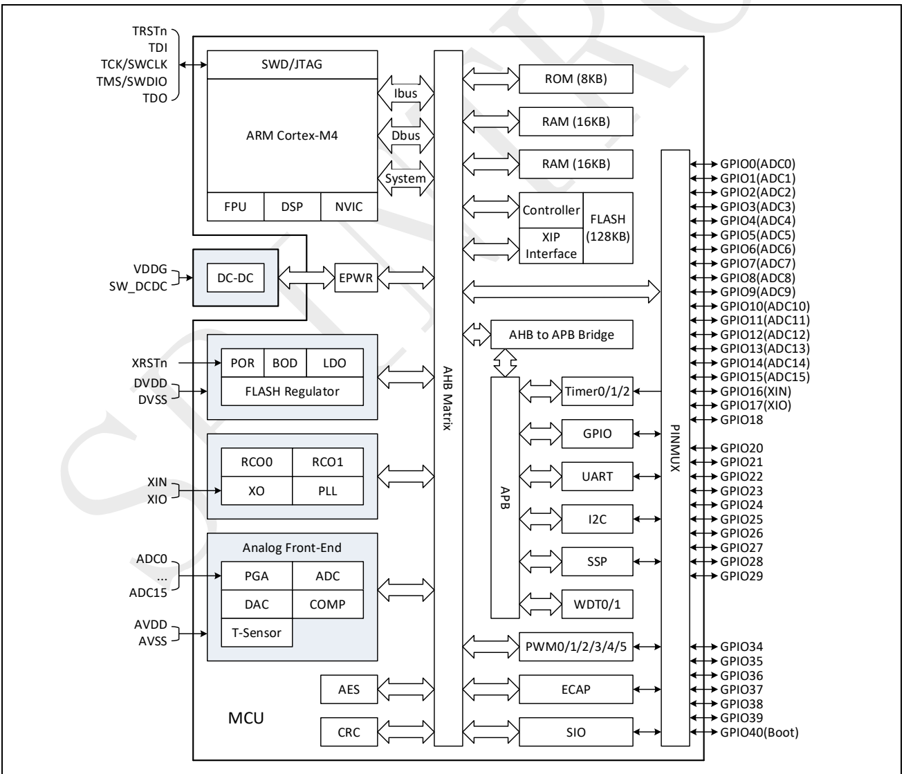
图 1-1: SPC1158 功能框图
