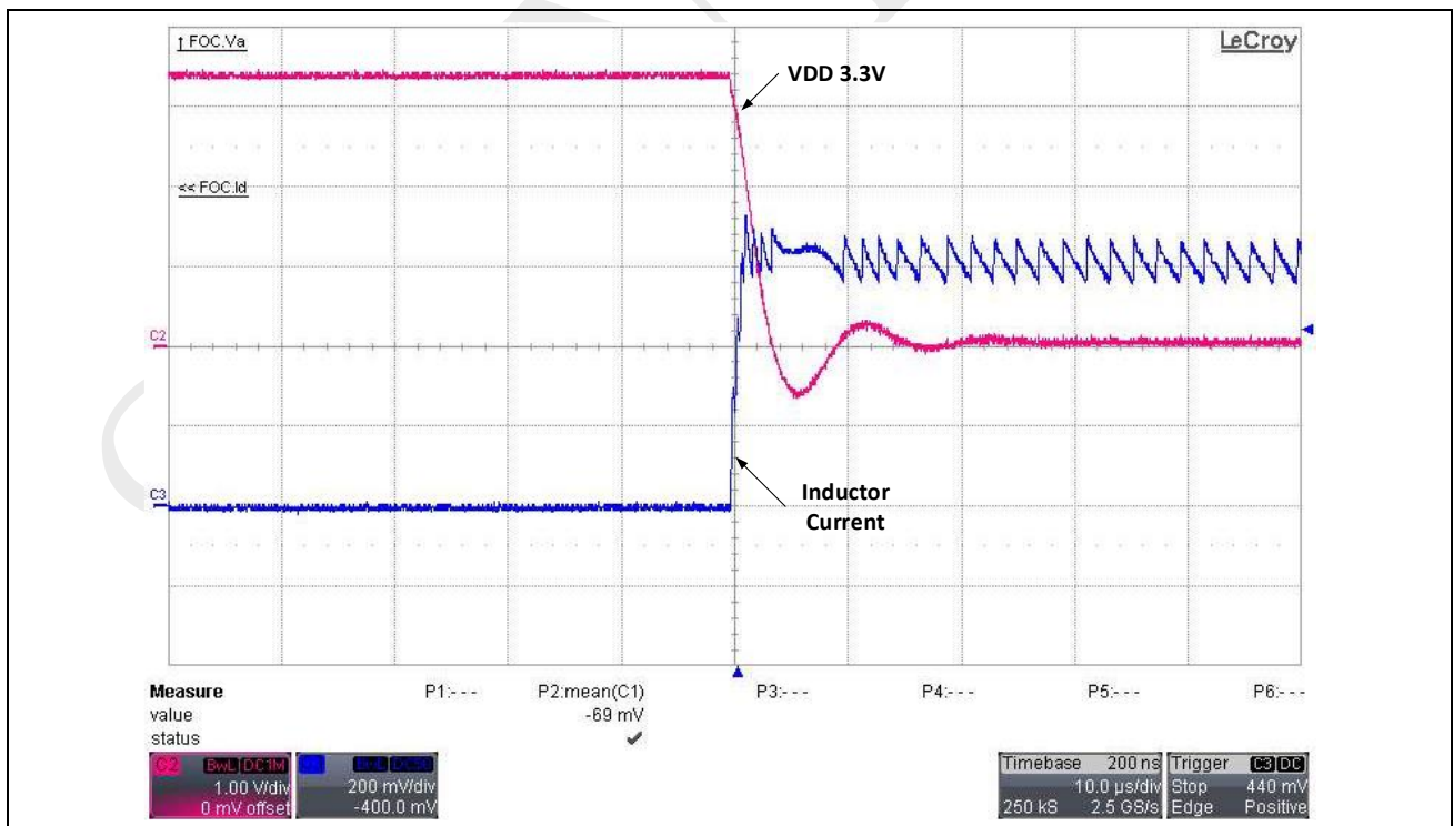
图 2-1：电感电流和电压变化
