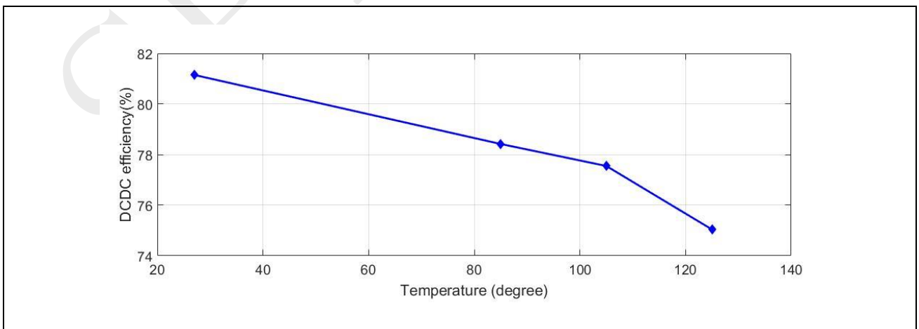
图 5-2: 开关电源效率随温度变化情况 (VDD33 负载电流为 500mA)
