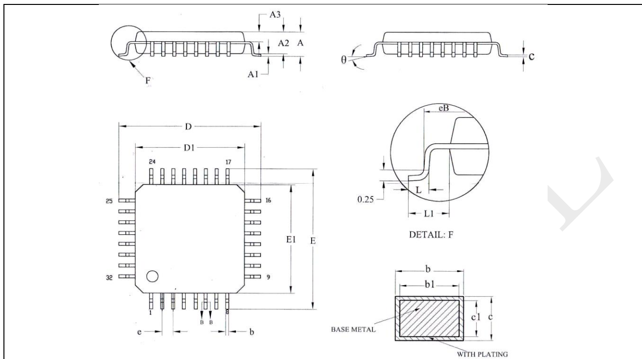
图 7-5: LQFP32 – 32 脚, 7 x 7 mm 薄型正方扁平封装图
