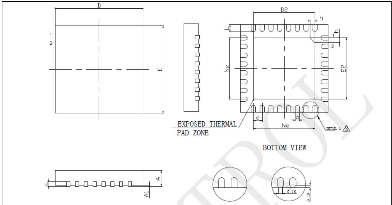
图 7-3: QFN32 – 32 脚, 5 x 5 mm 方形扁平无引脚封装
