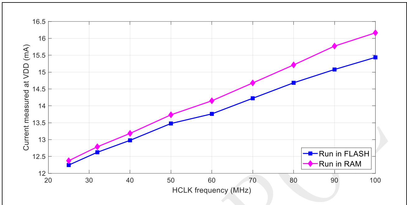
图 5-3: 典型工作电流随频率变化关系
