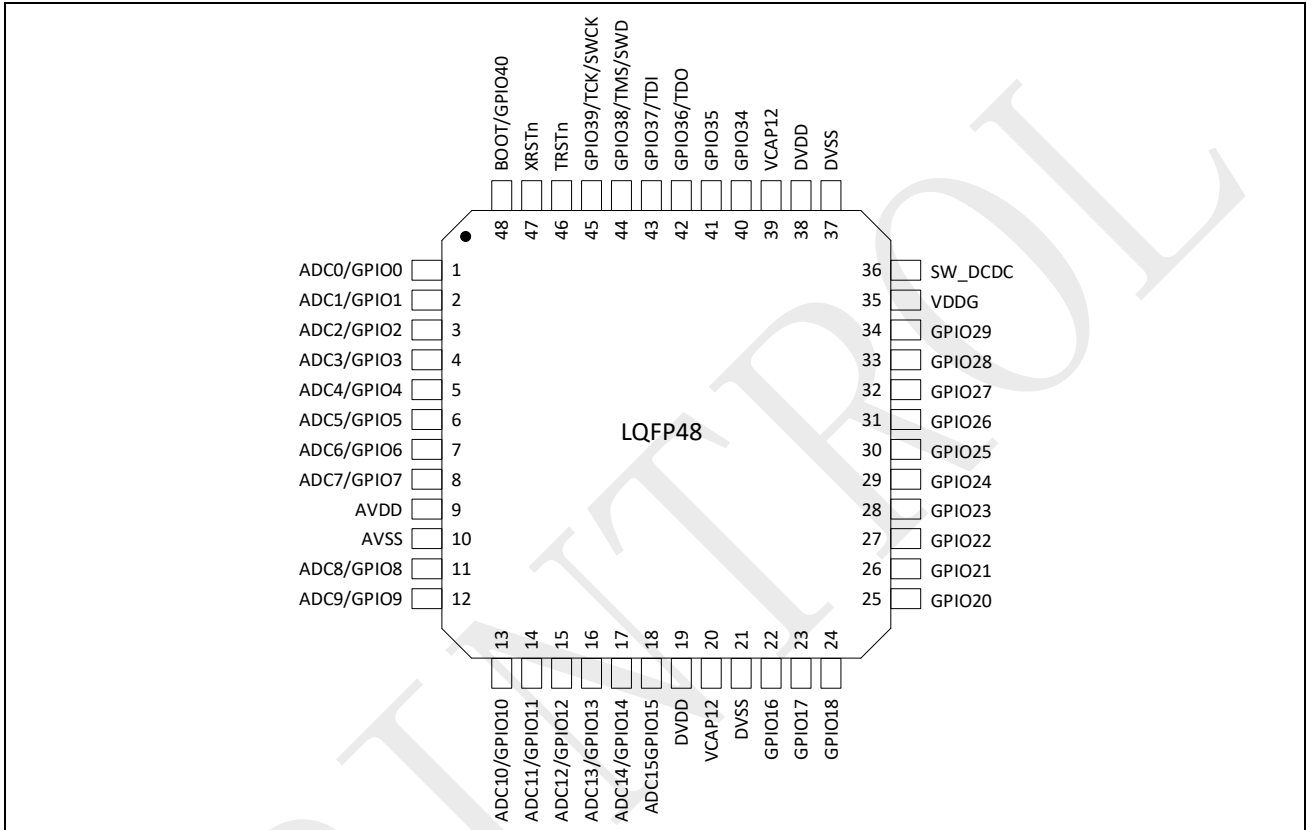
图 3-1: SPC1158 LQFP48 引脚排列
