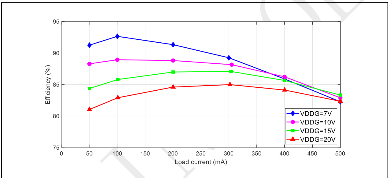
图 5-1: 开关电源效率 (TA = 25 °C)
