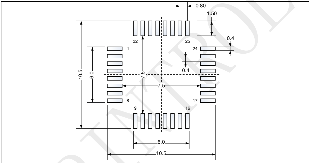
图 7-6: LQFP32 – 32 脚, 7 x 7 mm 薄型正方扁平封装建议尺寸
