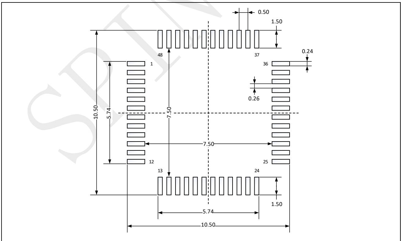
图 7-2: LQFP48 – 48 脚, 7 x 7 mm 薄型正方扁平封装建议尺寸
